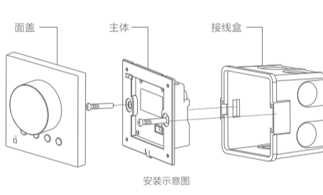
安装示意图
